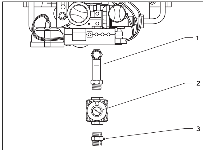
Рис. 4.1 Монтаж регулятора давления газа, тип RXi
